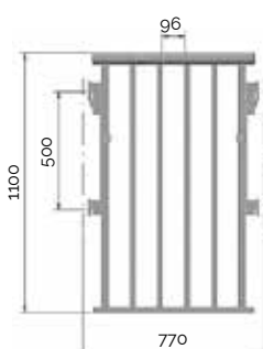
7053077 Skyddsräcke 1100/770 12,5 kg
