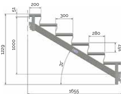
7102100 Vangstycke 1655x1000 24,0 kg
