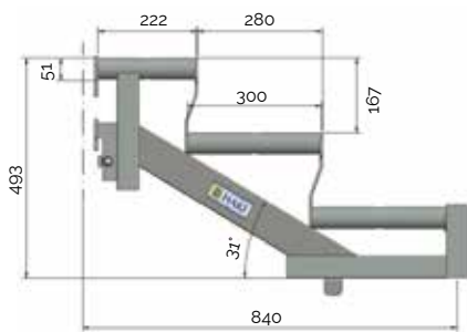
7102006 Vangstycke insteg 3 steg 10,7 kg
