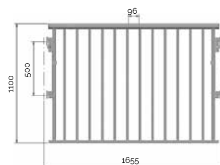
7053165 Skyddsräcke 1100/1655 23,0 kg
